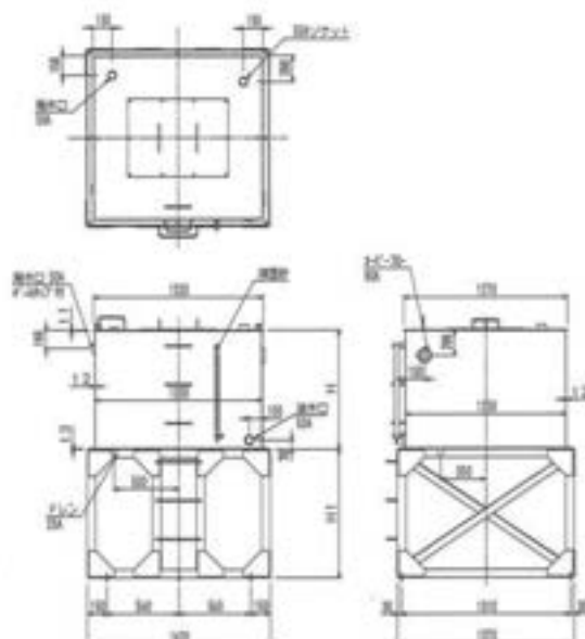
タンク容量：1000L、2000L
