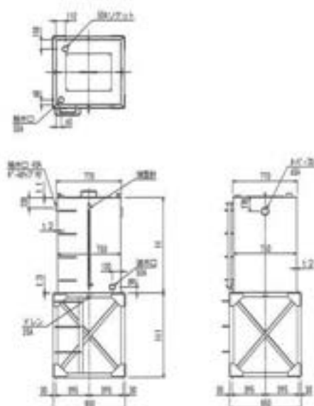
タンク容量：500L
